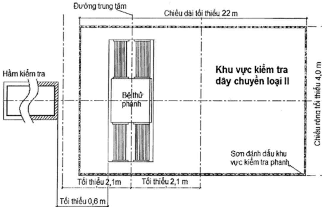
Hình 4. Khu vực kiểm tra phanh dây chuyên loại II
